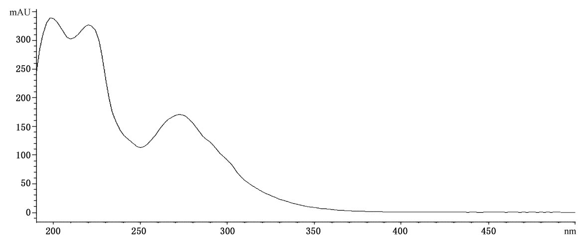
图 A.3 二硫化二苯并噻唑标准溶液的光谱图
